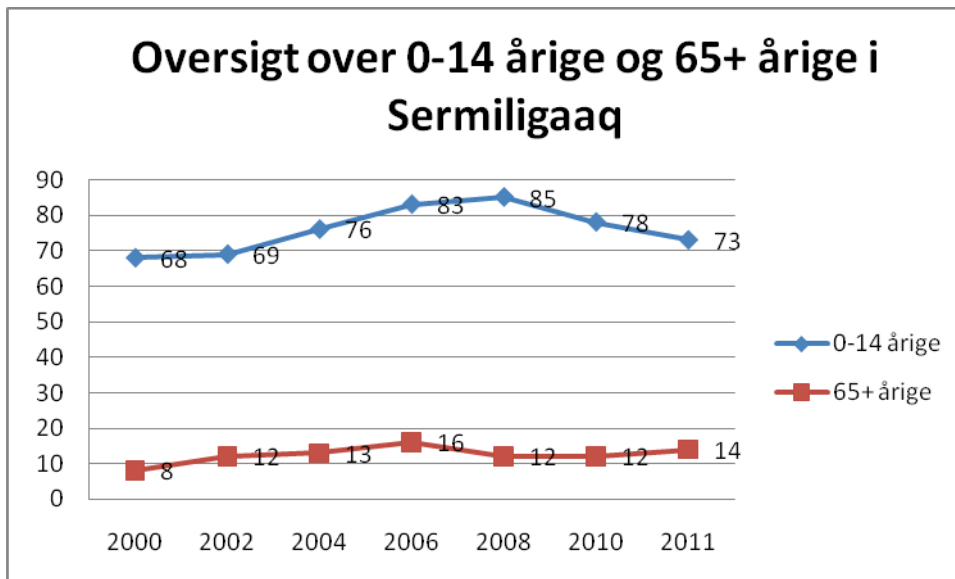
Figur 4. Forsørgerbyrde, Sermiligaaq
