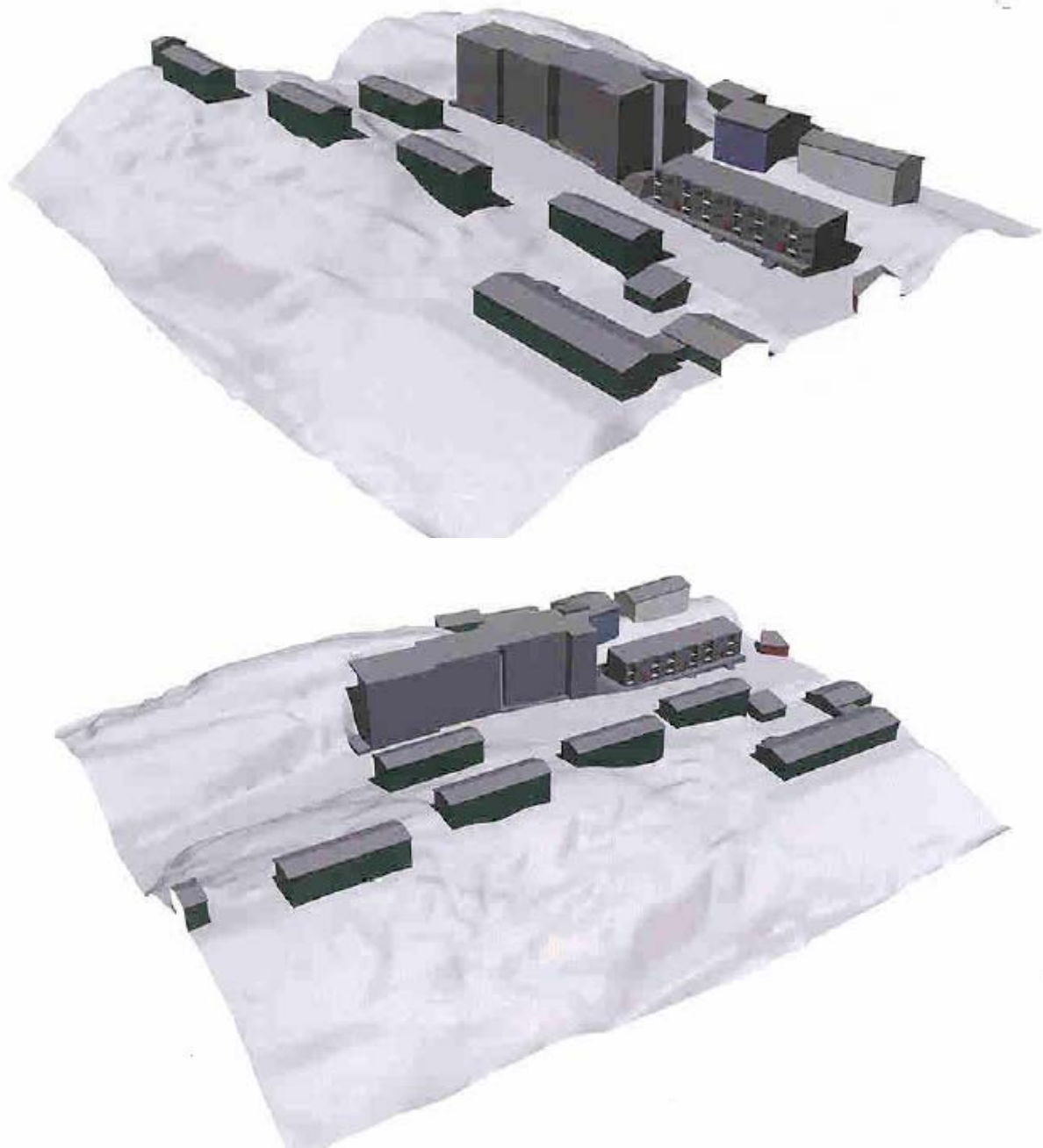
Asseq 3. Takussutissami sanaartorfissiani B1-imi aamma C1-imi kollegialiassatut sananeqartussatut siunnersuutigineqartoq angisuunn- gorlugu takutinneqarpoq. Qulaaniippoq immikkoortup avannaata kangianiit takutinneqarnera ataanilu immikkoortup kujataata kitaaniit takutinneqarnera..
