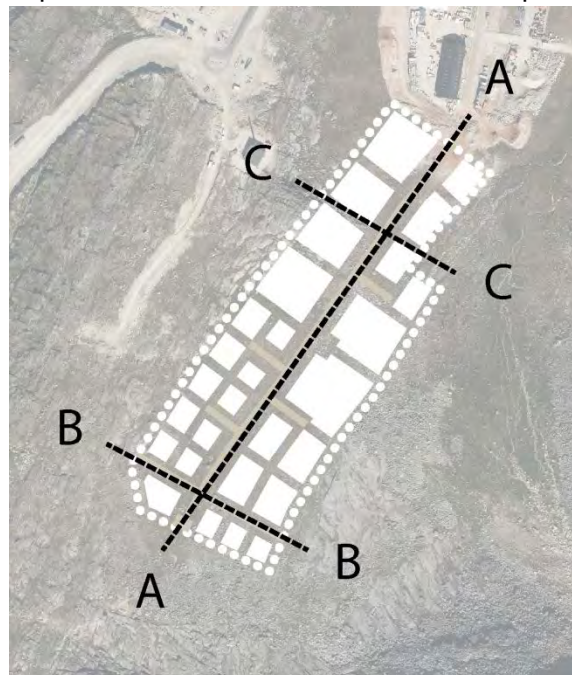
Fig. 7. Kommunimut pilersaarummut tapiliussami sanaartorfissat aqquserngillu..
